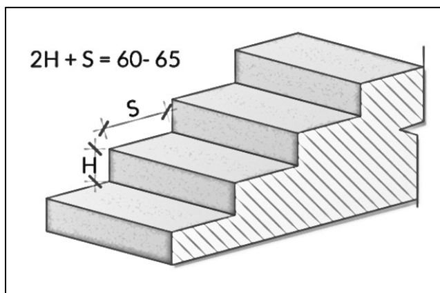
Obraz 73: Zależność między wysokością i szerokością stopni schodów
