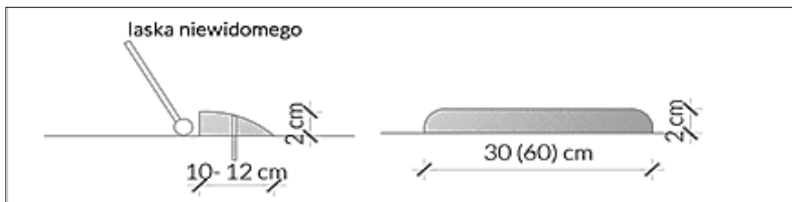
Obraz 72: Wygląd i parametry fakturowych oznaczeń nawierzchni typu D3
