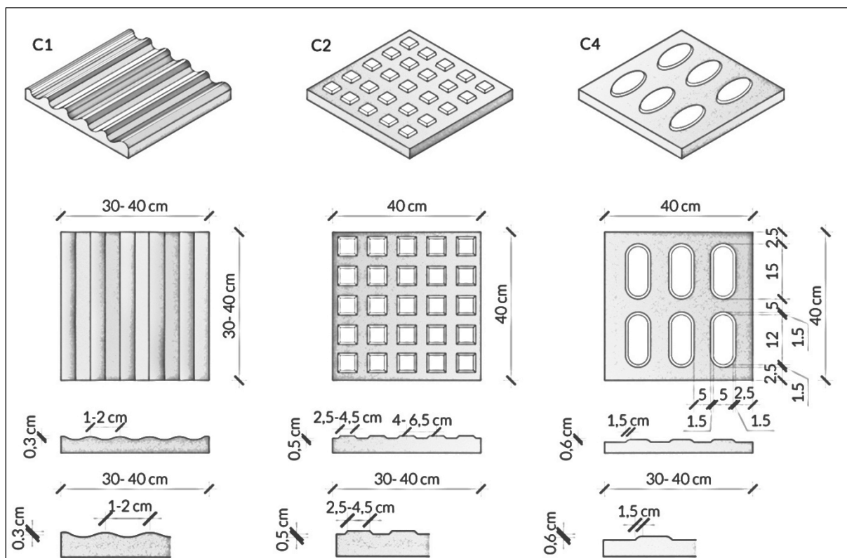
Obraz 71: Wygląd i parametry fakturowych oznaczeń nawierzchni typu C1, C2 i C4
