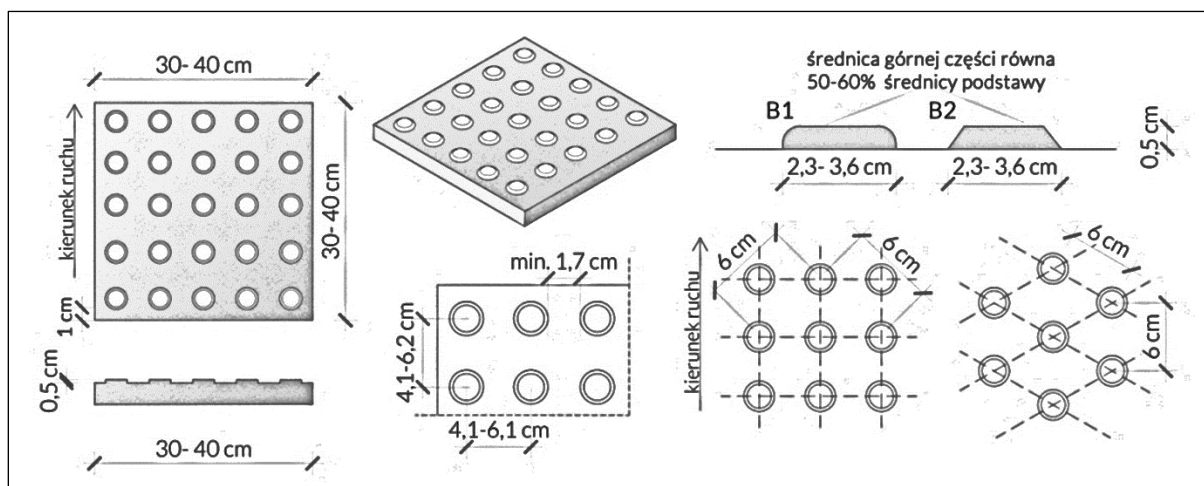
Obraz 70: Wygląd i parametry fakturowych oznaczeń nawierzchni typu B1 i B2
