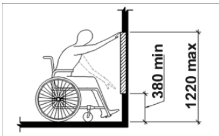
Obraz 65: Zasięg elementów obsługowych dla osoby poruszającej się na wózku
