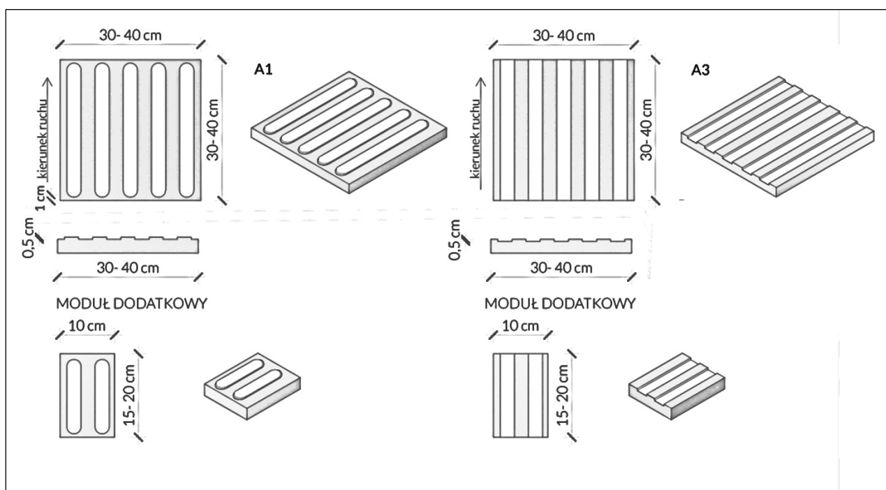
Obraz 69: Wygląd i parametry fakturowych oznaczeń nawierzchni typu A1 i A3
